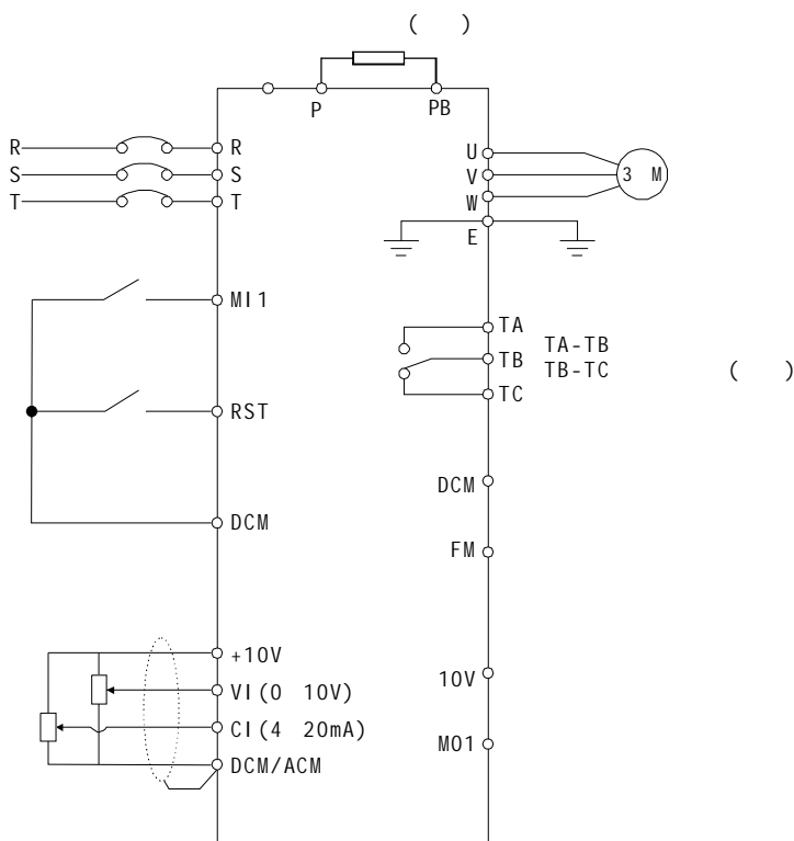
JTE286 基本配线图
